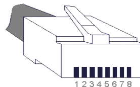
Abbildung 2: Anschlussbelegung RJ45 (IGC-konform)
