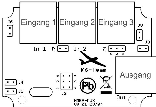
Abbildung 1: Anschlüsse
